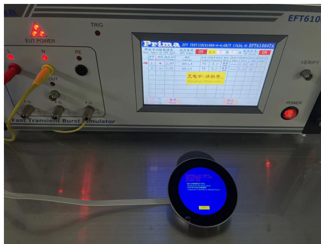
图 5-3 EFT 测试图
